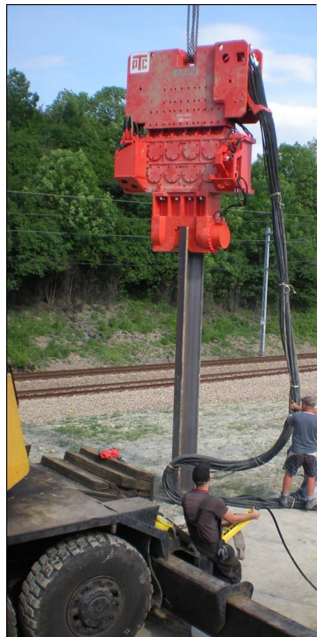
PTC 40HFV установлен в свободном подвесе на стреле мобильного крана Sennebogen. Вибропогружатель оснащен энергетической станцией PTC 900C с двигателем CAT C18 мощностью 571 кВт . Вибропогружатель укомплектован РВД с БРС и пультом радиоуправления.
