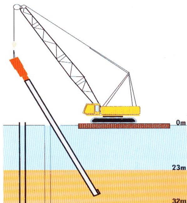
Вибропогружатель 120HDRK на погружении наклонных свай в г. Кобэ, Япония
